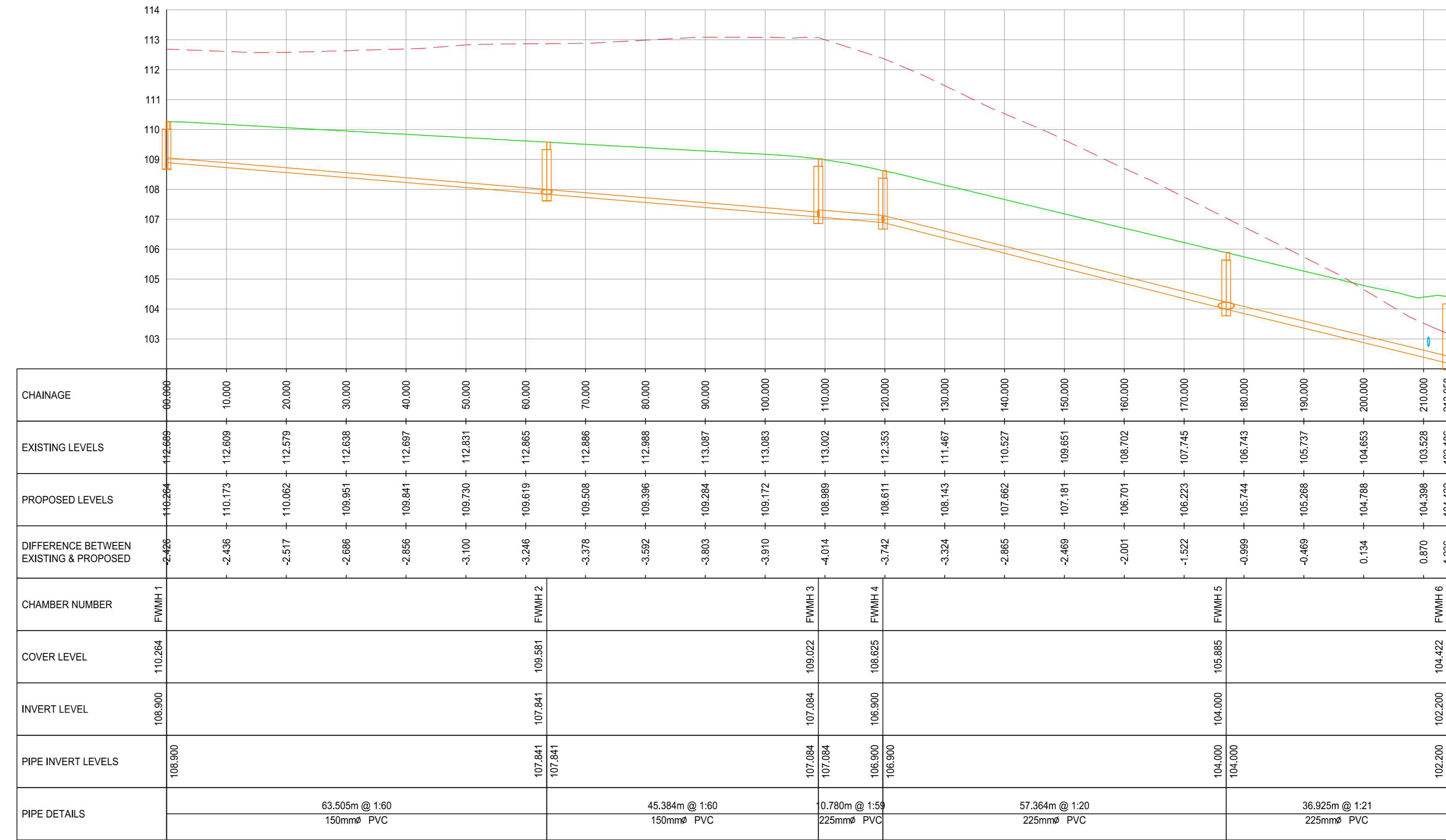
FW 2 SCALE: H 1:500, V 1:100. DATUM: 102.000
