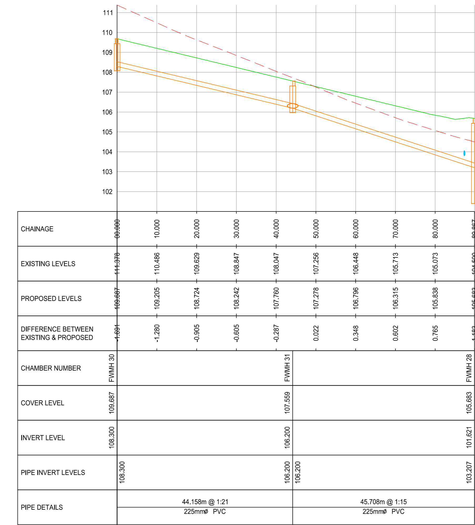
FW 5 SCALE: H 1:500, V 1:100. DATUM: 101.000
