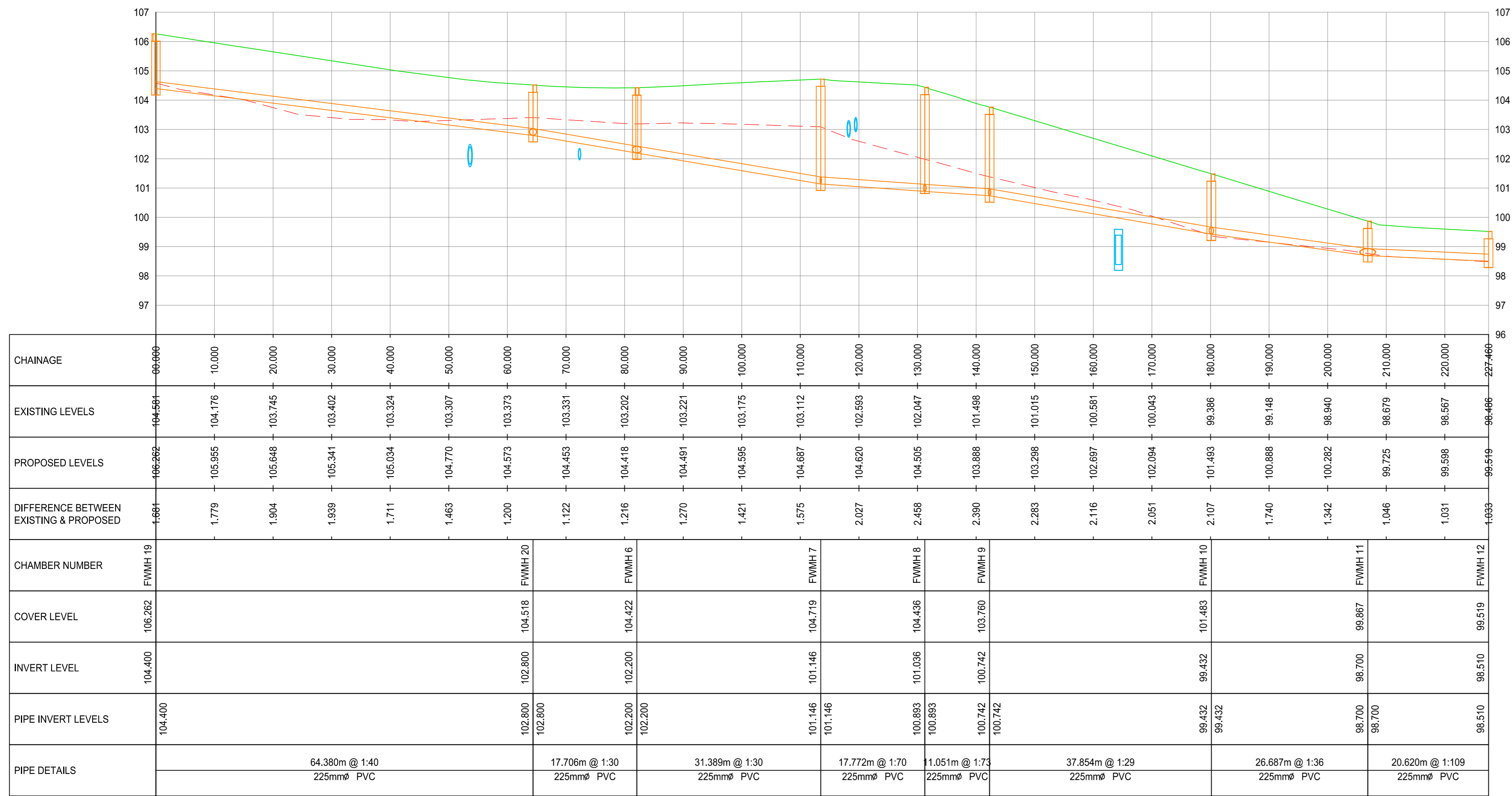
FW 1 SCALE: H 1:500, V 1:100. DATUM: 96.000
